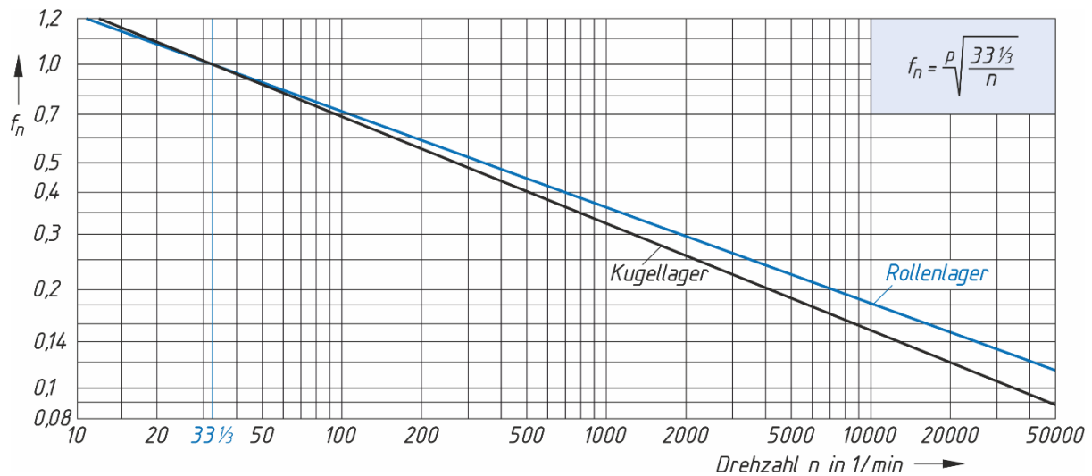
TB 14-4 Drehzahlfaktor f_n für Wälzlager
