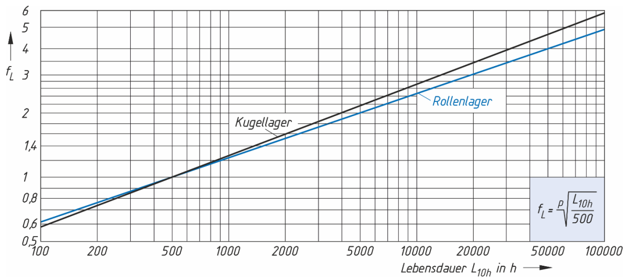
TB 14-5 Lebensdauerfaktor f_L für Wälzlager
